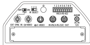
BRC-300
